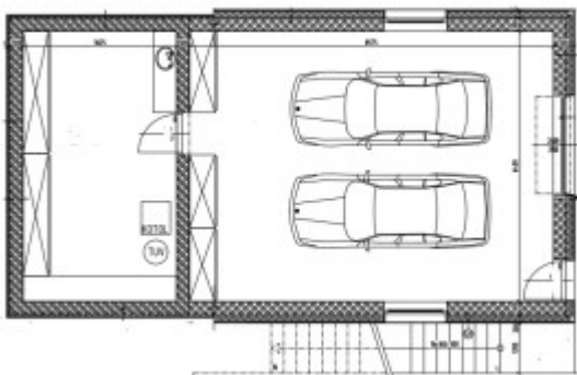
Pôdorys : Suterén
