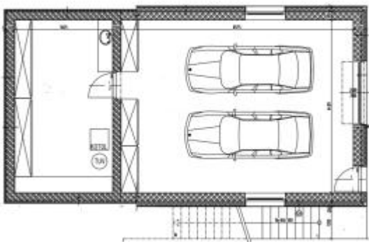
Pôdorys : Suterén
